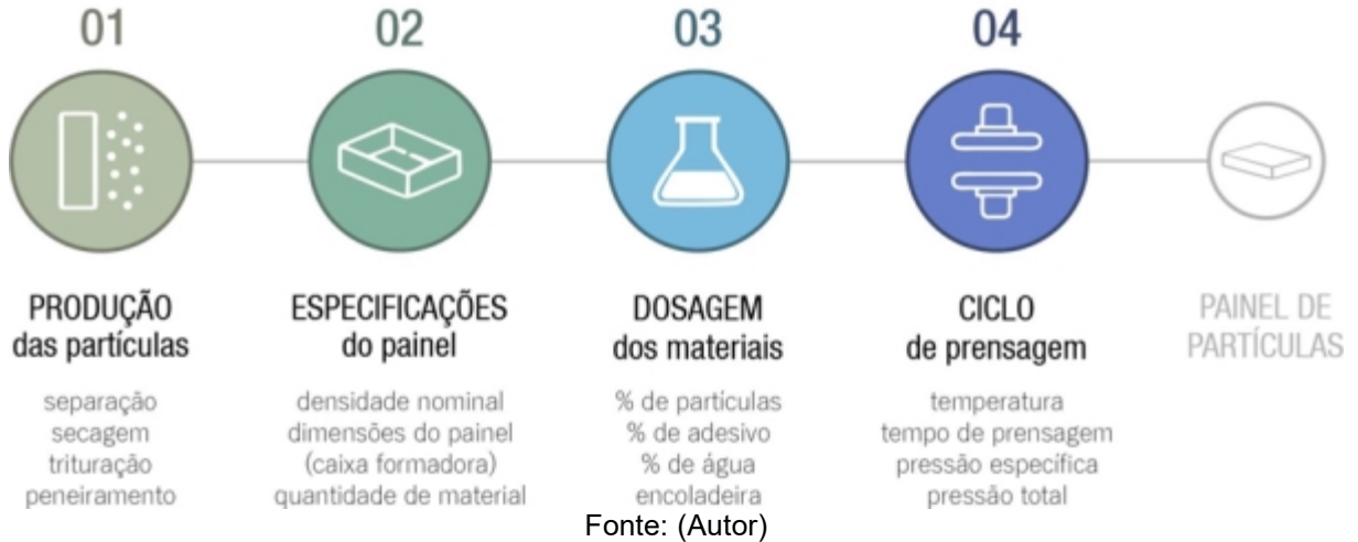
Figura 3. Metodologia para a produção de painéis de partículas.
